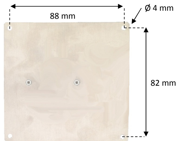
Vue de la plaque de fixation
